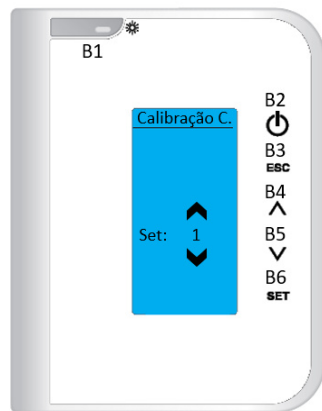
Acéder ao Menu Calibração Cóclea
