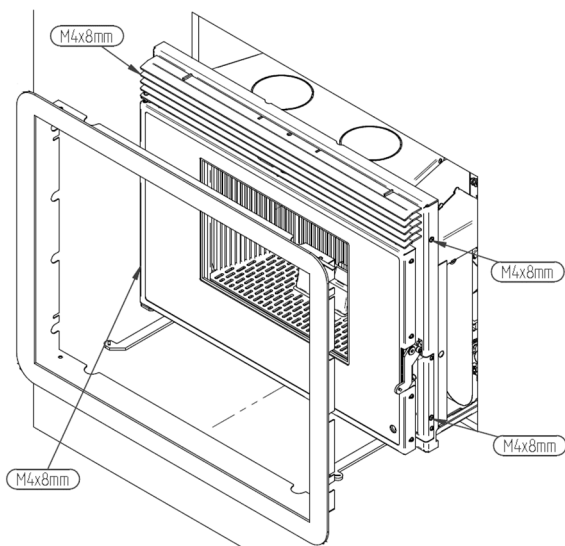
Figura 37 – Demonstração dos elementos de ligação da moldura
