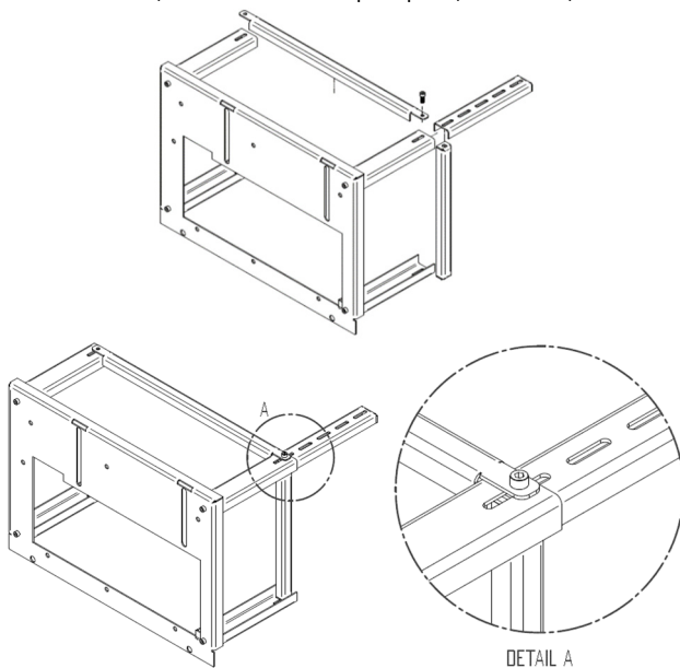
Figura 32 – Montagem mesa auxiliar
