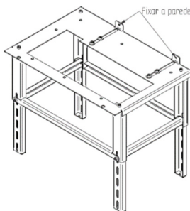
Figura 36 – Montagem mesa auxiliar
