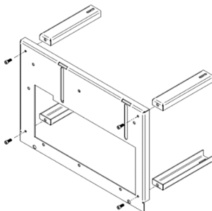
Figura 31 – Montagem mesa auxiliar
