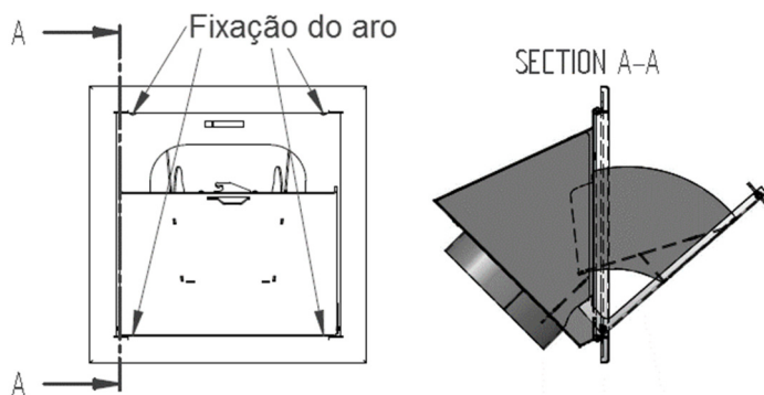
Figura 19 – Instalação equipamento
