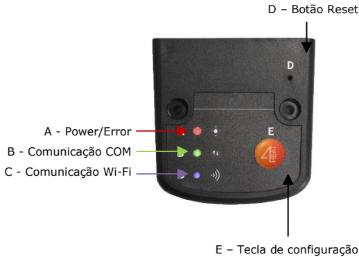
Figura 5 – Módulo Wi-Fi
