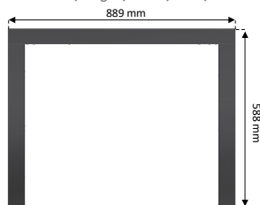
Moldura 3 lados 50mm / Moldura 3 lados de 50mm / 3 sided 50mm frame / Cadre 3 côtes de 50mm / Telaio 3 lati 50mm
